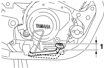
1. Bromspedalens spel
