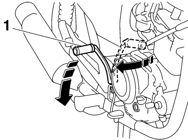
1. Startkick
