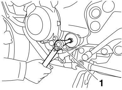
1. Momentnyckel
