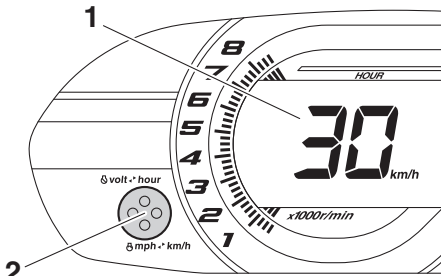
1 Ταχύμετρο
