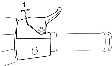
1 Τζόγος χειρόγκαζου
