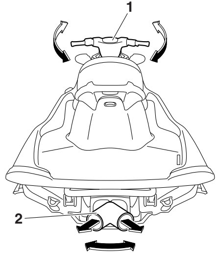
1 Χειρολαβές τιμονιού
