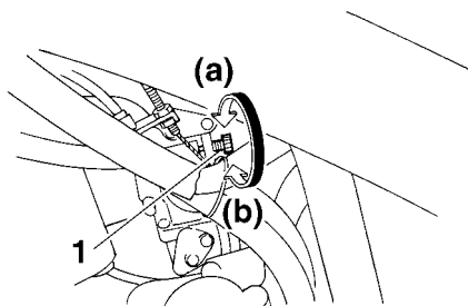
1. Tomgångsskruv
